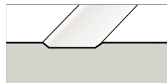
Nordic – Querschnitt Türblatt mit vertieften Profilen
